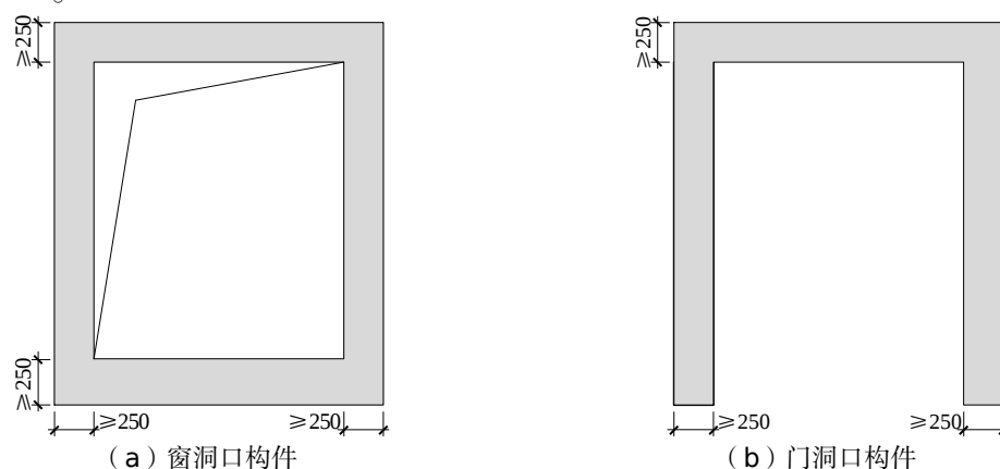
图 8.2.2 带洞口预制空心墙板尺寸要求示意
