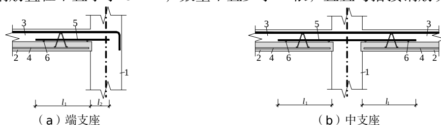
图 6.4.4 预制底板纵向受力钢筋不伸入支座构造示意图
