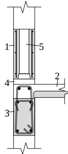
图 8.3.5 窗下墙连接构造示意
