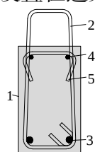
图 8.2.4 叠合梁构造示意
